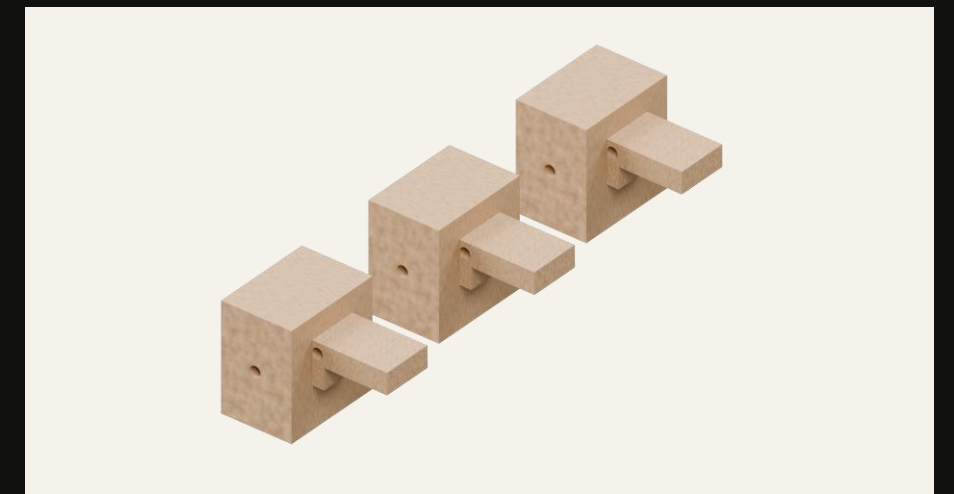
G / Tres garfios · unión principal
