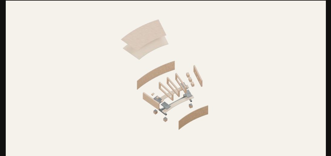
Despiece de módulo
