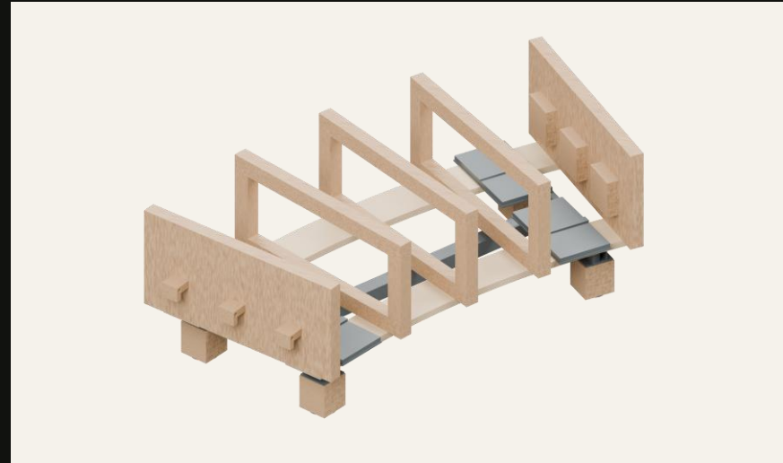
I longitudinal · marcos de listones
