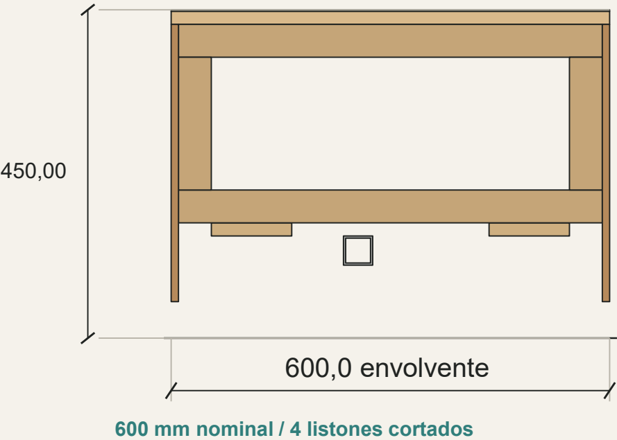
A-A / costilla central
