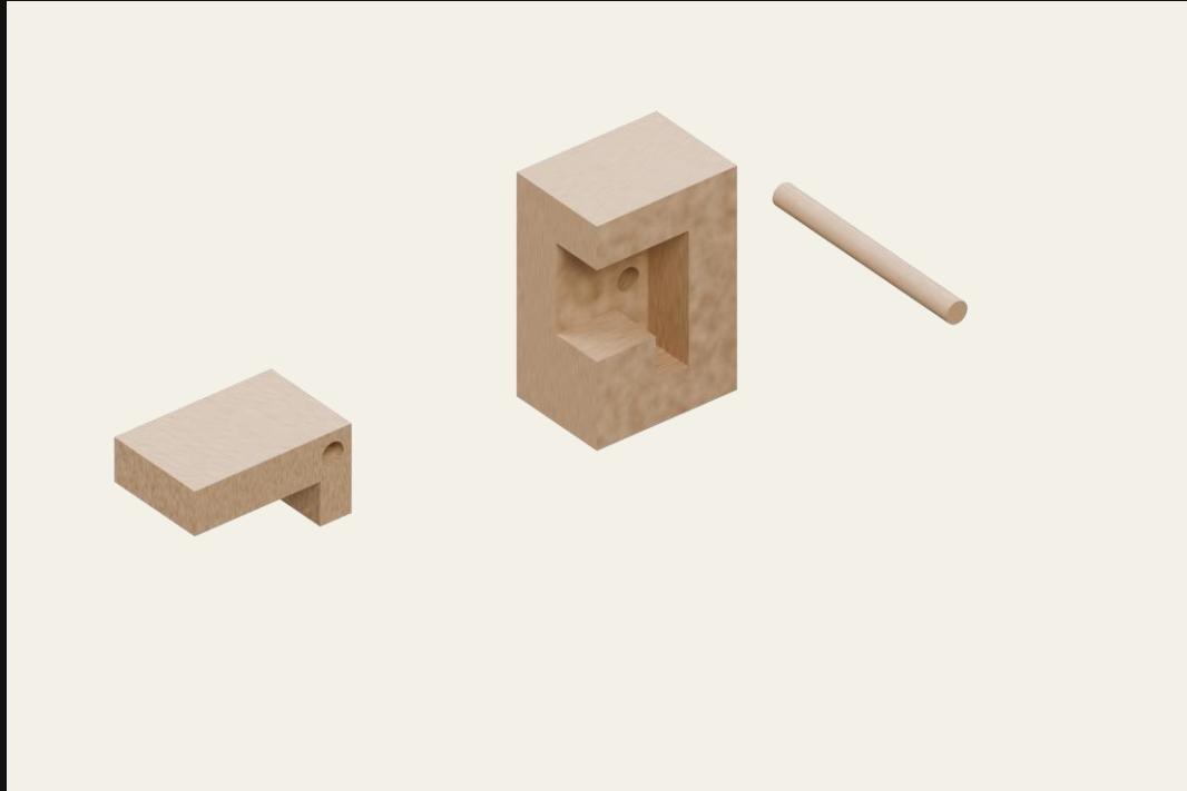
G / garfio, receptor y seguro · despiece
